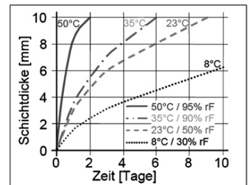
Diagramm 1: Durchhärtegeschwindigkeit von 1-Komponenten Sikasil®
